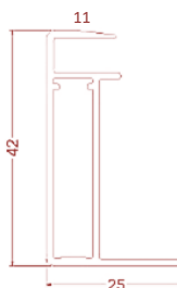
Vue en coupe du cadre, champ long
