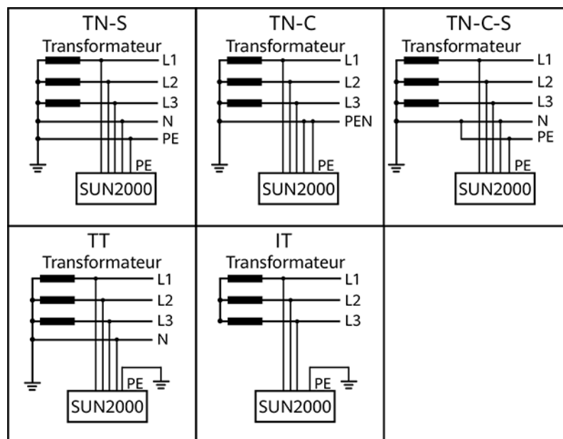
Figure 2-5 Réseaux électriques pris en charge
